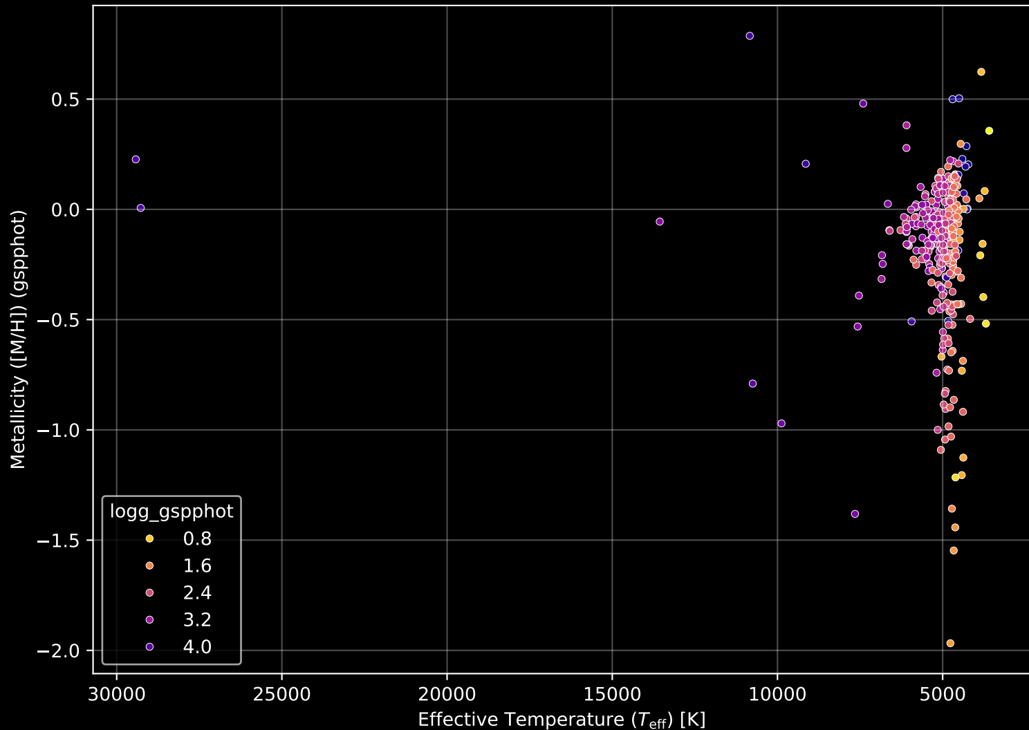
APOGEE DR17 Field: [214+00] Stellar Population Parameters (n= 377)
